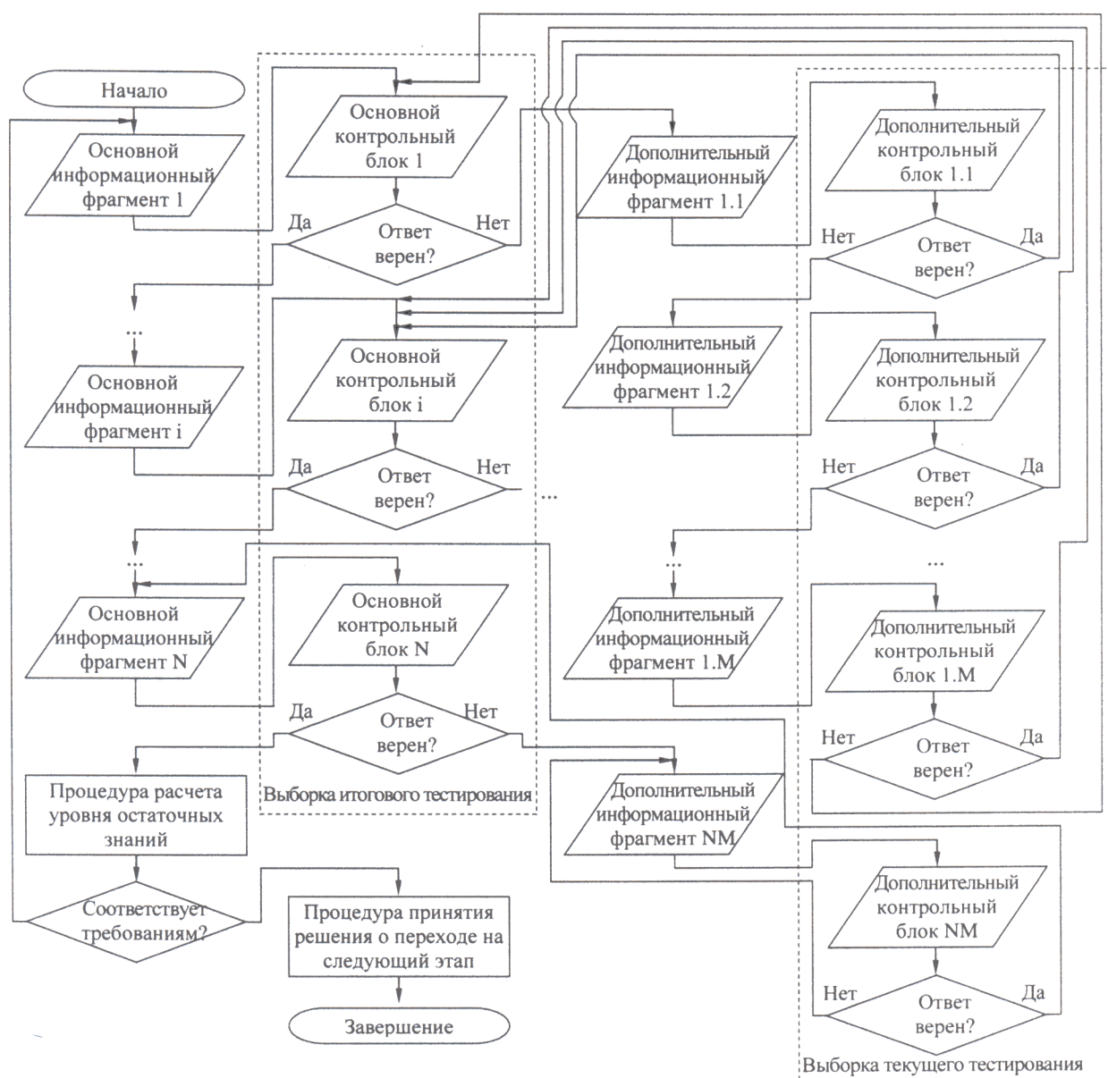
Рис. 3. Алгоритм отображения информационных фрагментов и контрольных вопросов основного и дополнительного блоков
