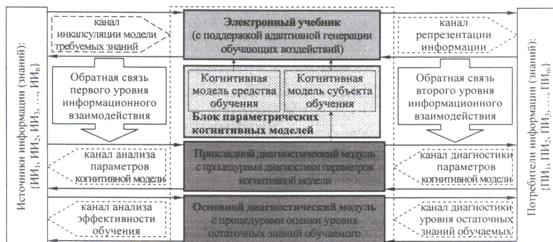
Рис. 1. Структурная схема системы автоматизированного обучения со свойствами адаптации на основе блока параметрических когнитивных моделей
