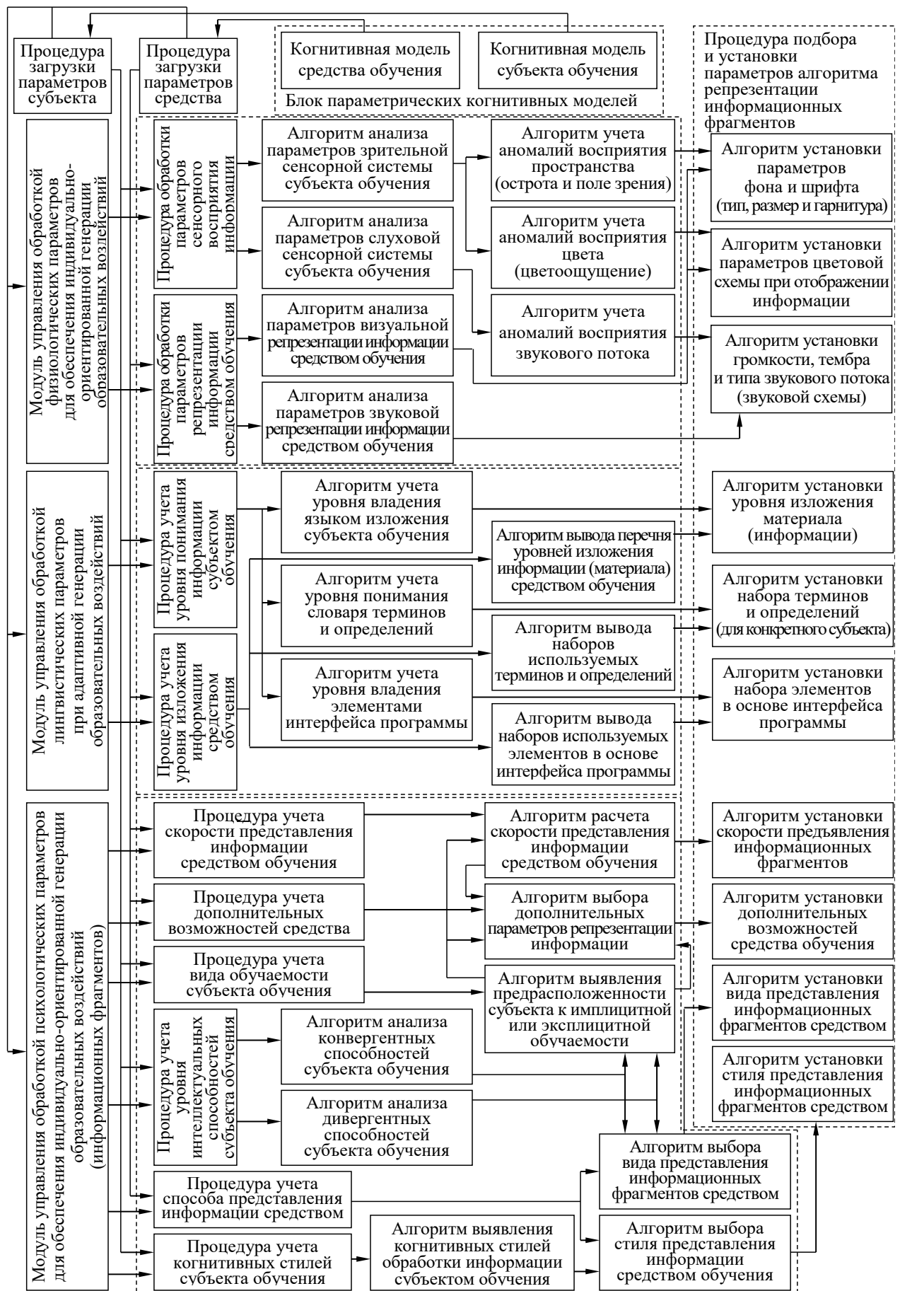
Рис. 3. Структура процессора адаптивной репрезентации информационных фрагментов
