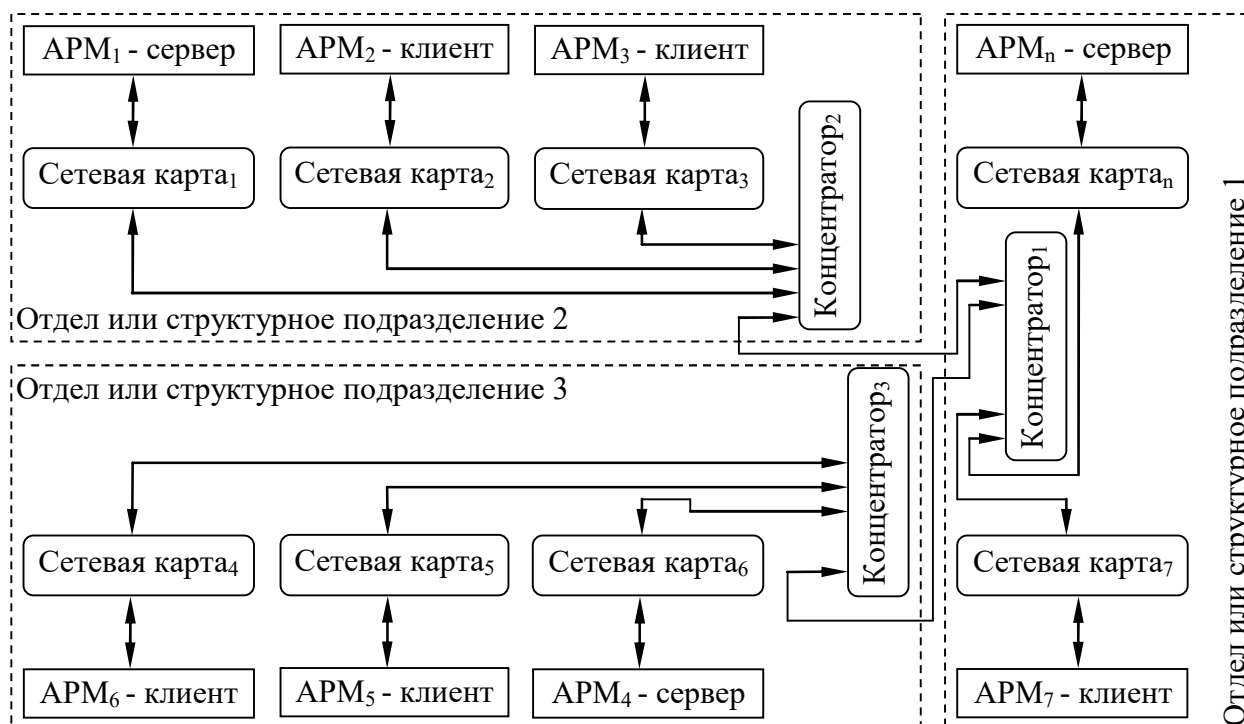
Рис. 2.10. Топология локальной вычислительной сети типа «кольцо-звезда»
